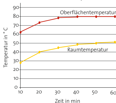
Schnelle Erwärmung der Heizelemente und der Raumtemperatur
